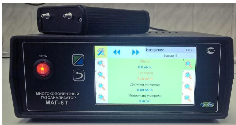
Рисунок 6 – Внешний вид газоанализатора МАГ-6 исполнения МАГ-6 Т-8 (с одним внешним измерительным преобразователем МАГ-6)
